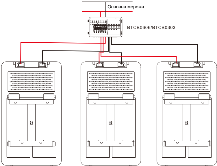
Рисунок 1: Паралельне підключення трьох акумуляторних блоків
